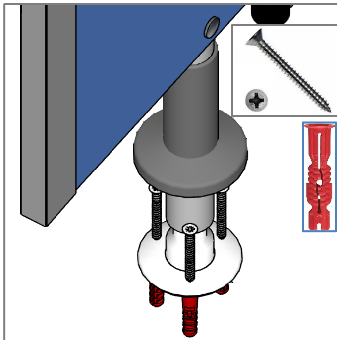
Stelpoot Aluminium met kunststof Sok Schroef 4,2x 38 DIN 7982 PH (verzonken kop) Universeelplug HUD-2 6x30
