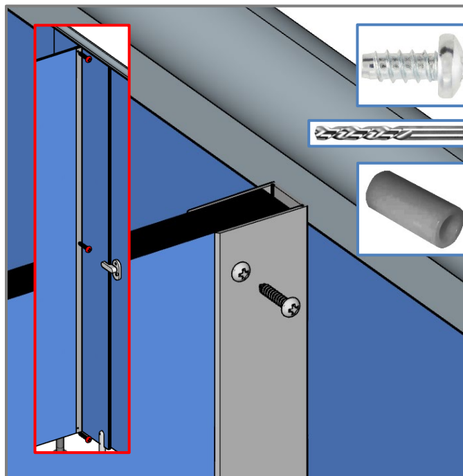
U-Profiel aan de tussenwand
