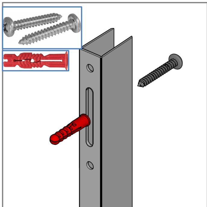
Aluminium U-Profiel 17x30mm op de muur Schroef DIN 7981-C 4,8x38 A2 (PH2) (bolkop) Universeelplug HUD-2 6x30 Steenboor Ø6mm
