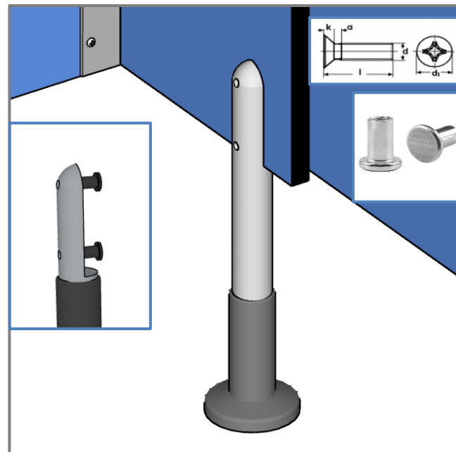
Stelpoot Aluminium met kunststof Sok DIN 965 M5x20 A2 (PH2) Blinde busmoer RVS A4 M5 x 11
