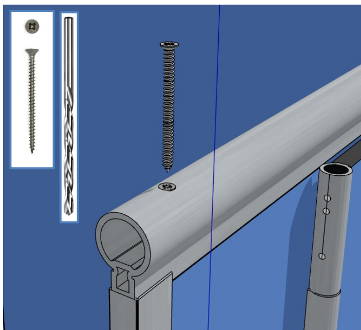
Koppelprofiel Aluminium Schroef Spaanplaat Schroef 4.0x60 A2 (PZ2) HSS spiraalboor Ø3.6mm DIN 340 type 510 Vorboren met boor Ø 3,6 mm
